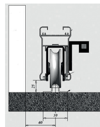
Galets avec renforts de fixation pour crémaillère
